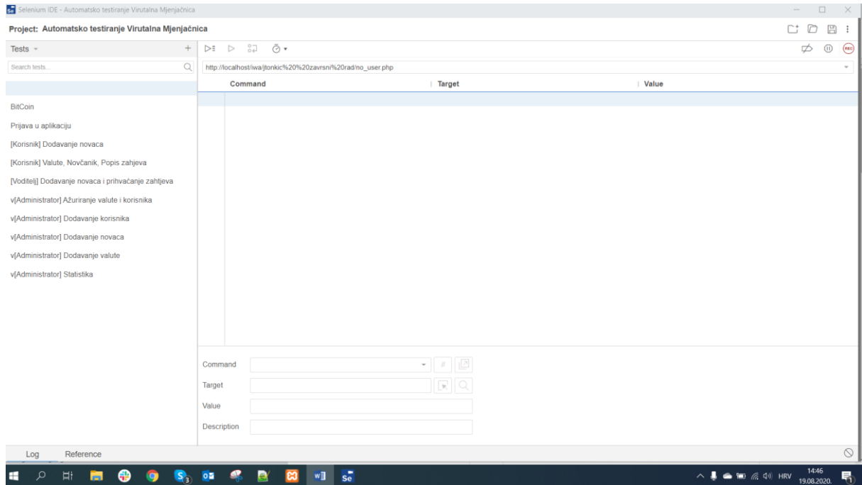
Slika 17. Selenium IDE
