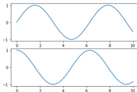
Slika 2: Rezultat vizualizacije sinus i kosinus funkcija
