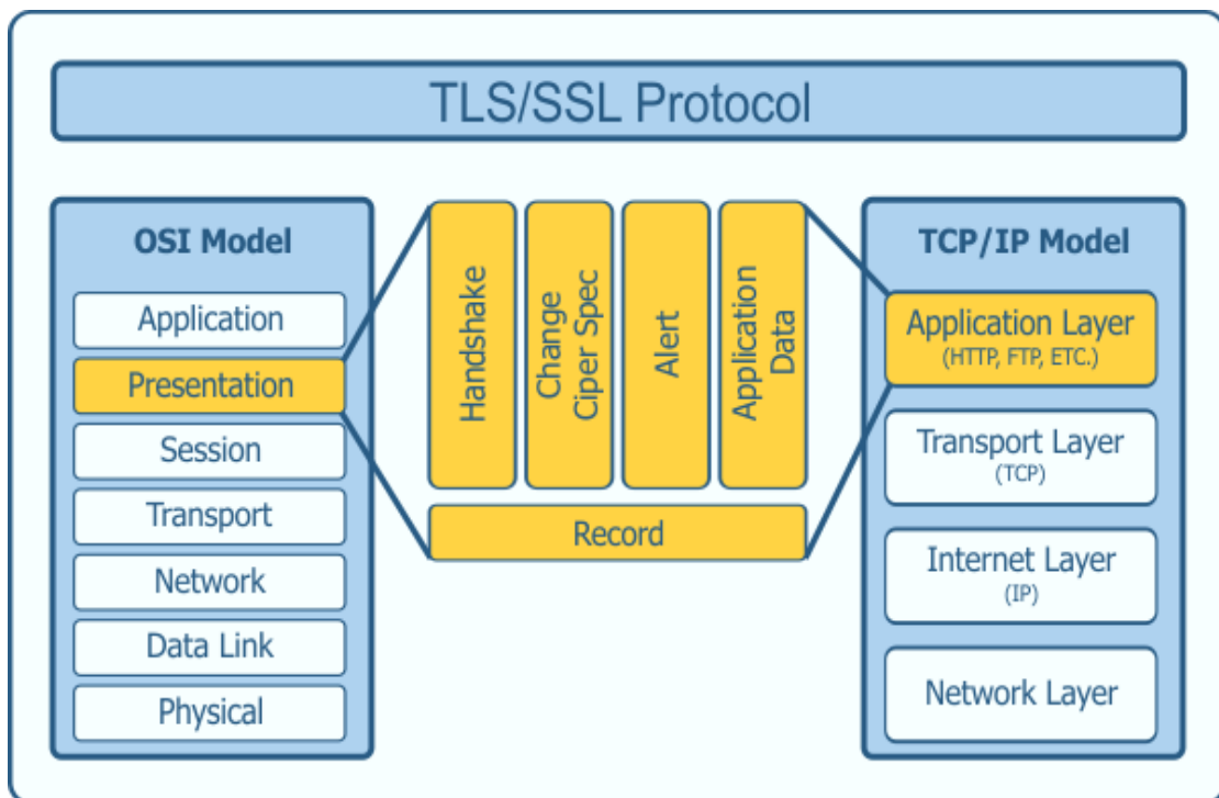
Slika 1: Prikaz SSL/TLS protokola unutar mrežnih modela OSI i TCP/IP [2]
