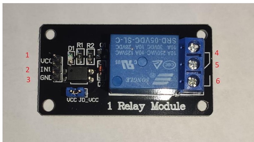
Slika 5. Korišteni relej s označenim ključnim dijelovima
