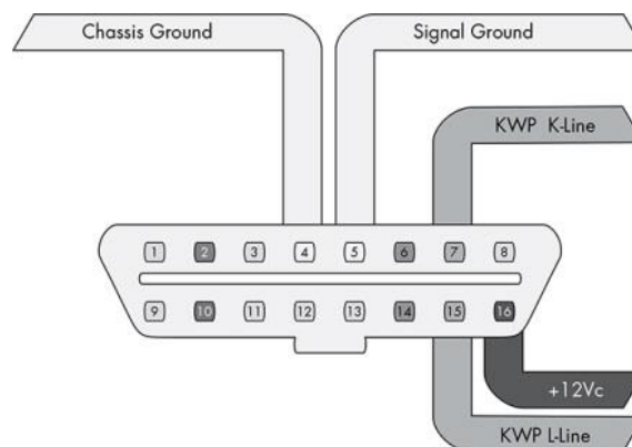
Slika 6: ISO 9141-2 pinout
