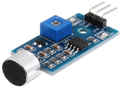
Slika 41. Mikrofon
