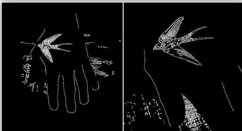
Slika 12: Detekcija rubova
