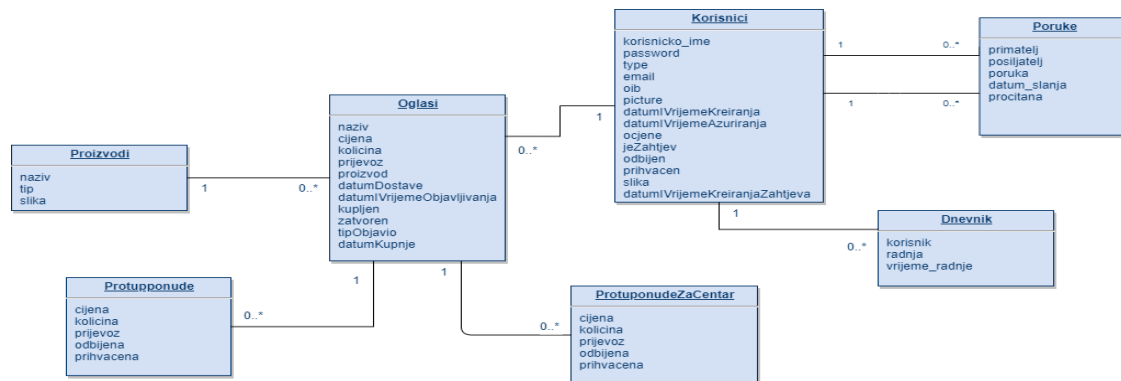
Slika 6: UML dijagram konceptualnog modela podataka (Izvor: autorski rad)
