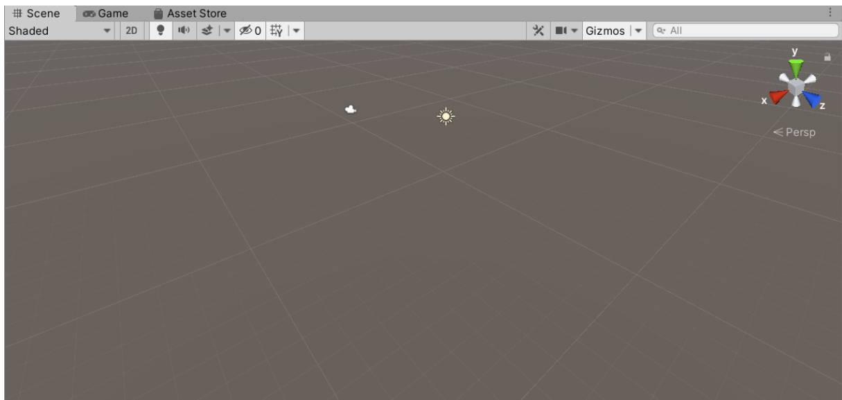
Slika 2: Scene view
