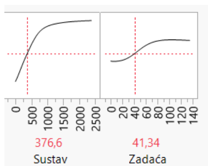
Slika 25: Prediction profiler [izrada autora]
