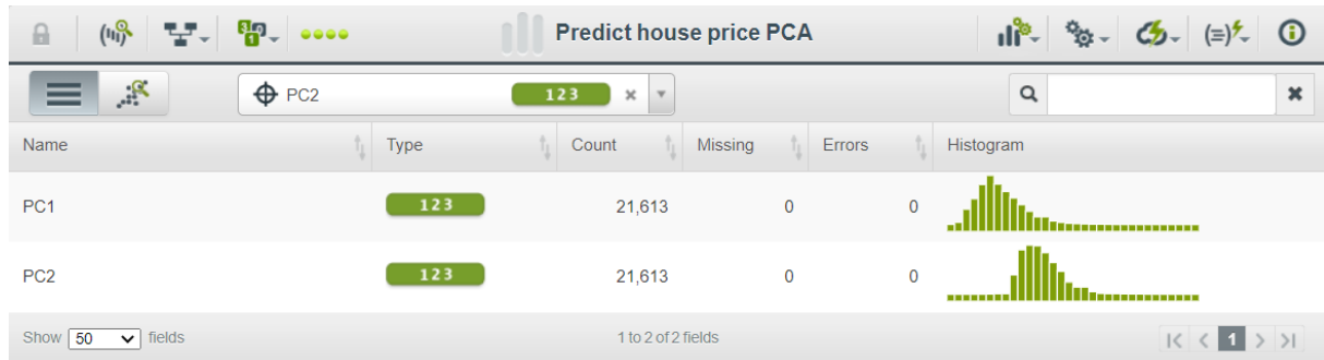
Slika 13: Skup podataka dobiven analizom glavnih komponentata (Izvor: vlastita izrada)
