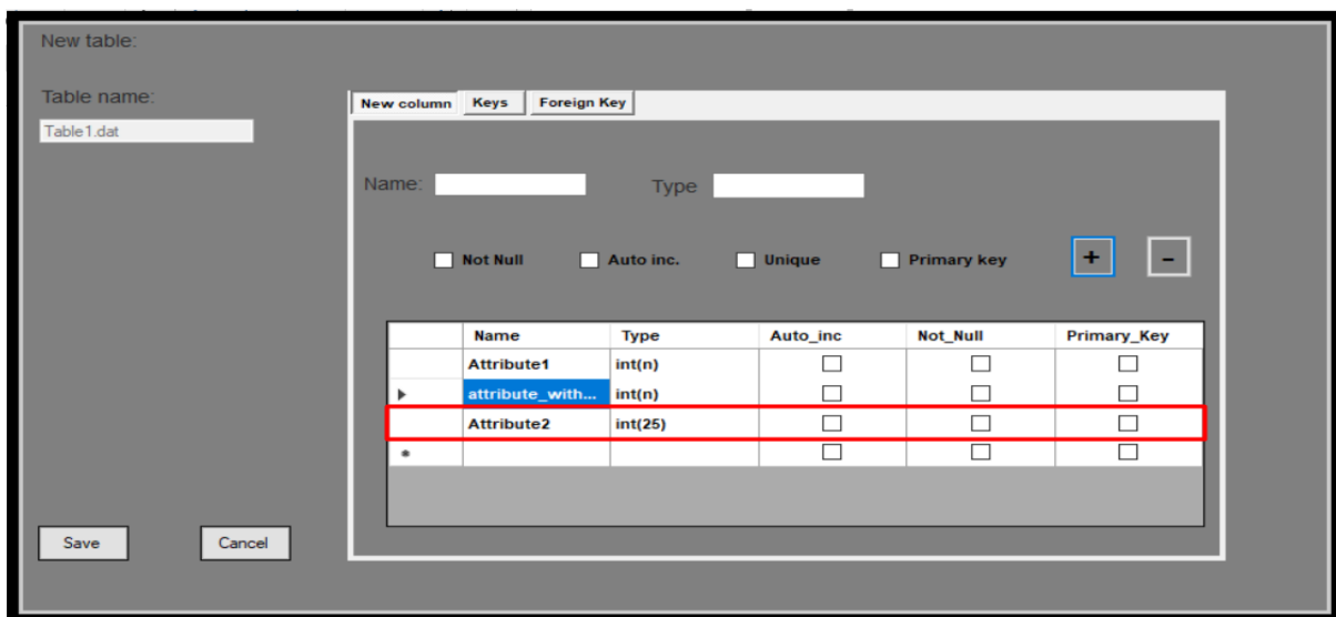
Slika 32: Unos tipa podataka sa određenom veličinom (Izvor: vlastita izrada)
