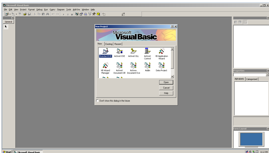
Slika 2: Visual Basic 6 [4]
