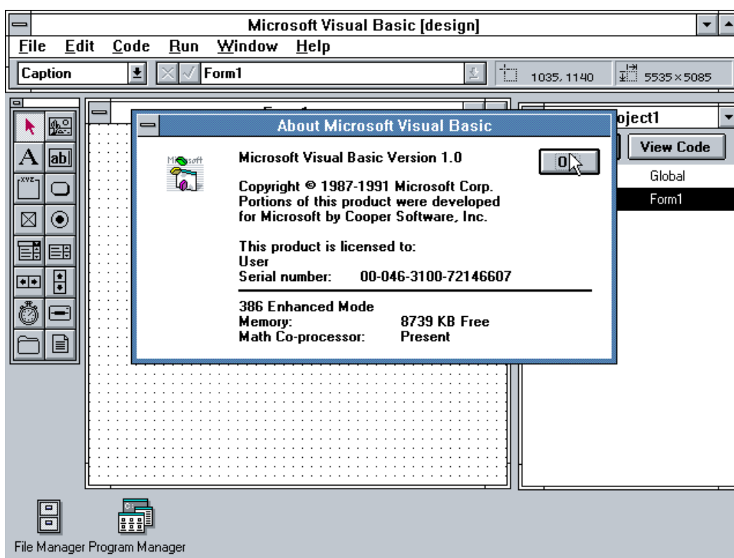
Slika 1: Visual Basic 1.0 [3]
