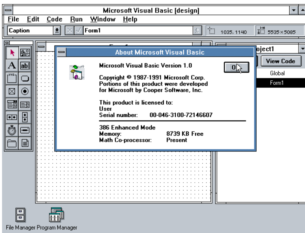
Slika 1: Visual Basic 1.0 [3]
