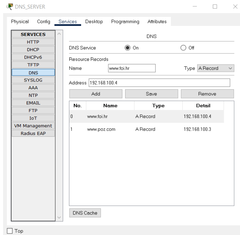
Slika 21: Postavljanje DNS servisa [Autorski rad]
