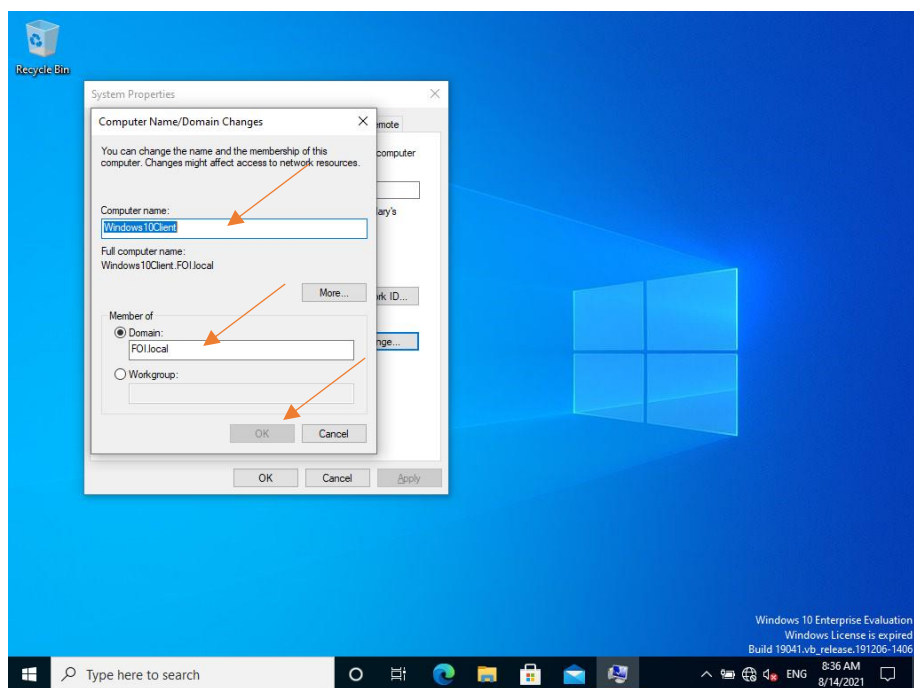
Slika 51 Član domene
