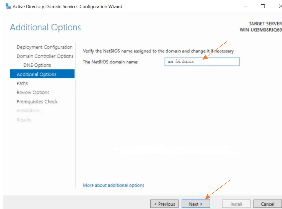
Slika 33 NetBios
