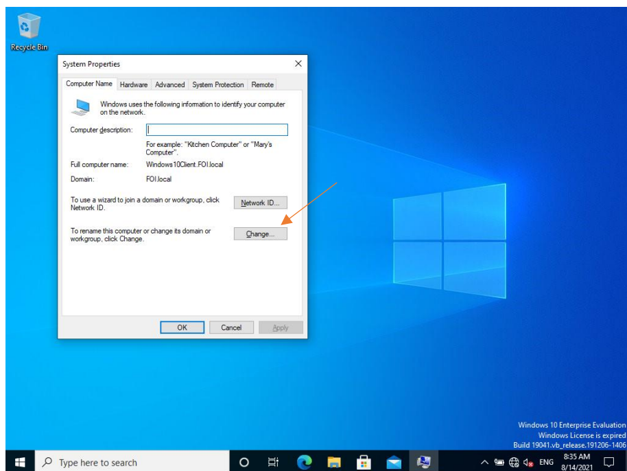
Slika 50 Postavke sistema 2
