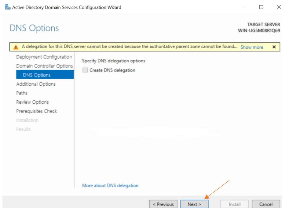
Slika 32 DNS opcije
