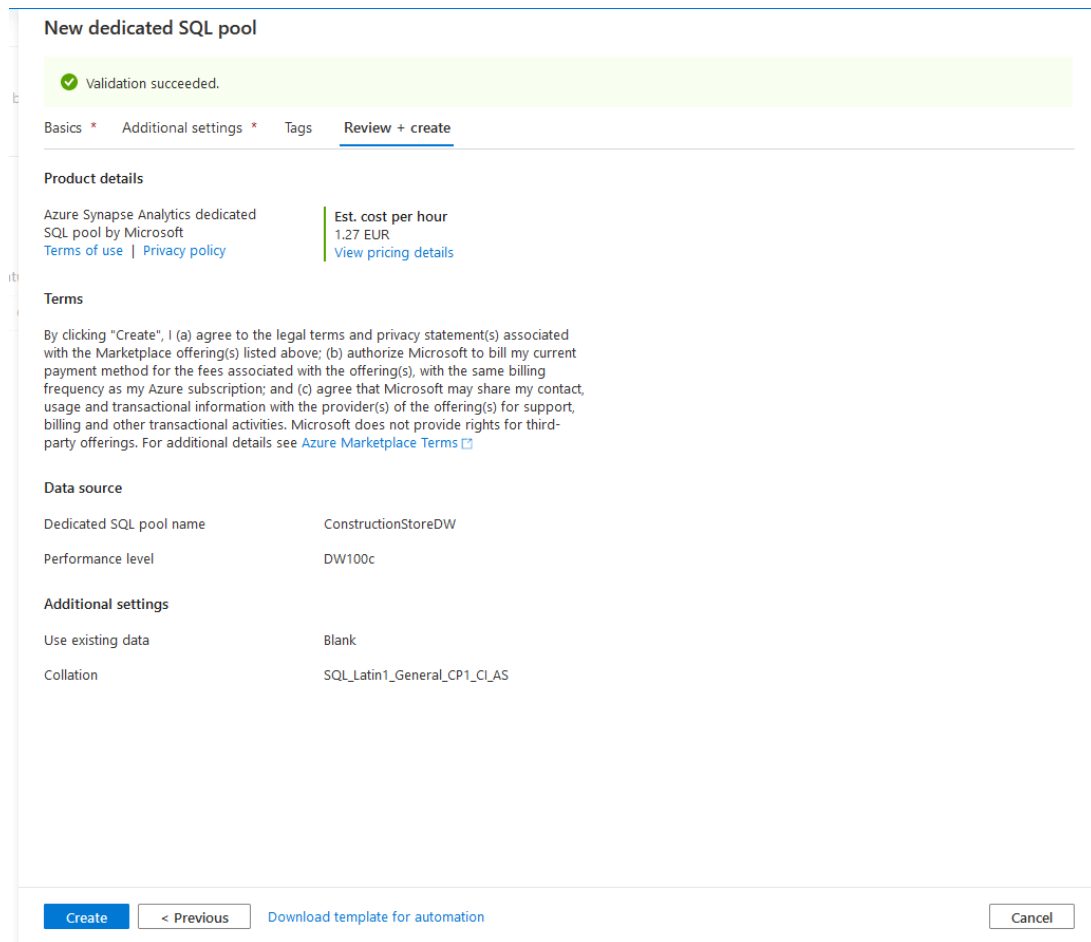
Slika 20: Kreiranje SQL bazena (skladišta podataka) za Synapse(2)
