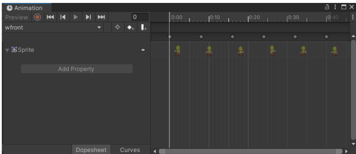
Slika 4. Animation prozor
