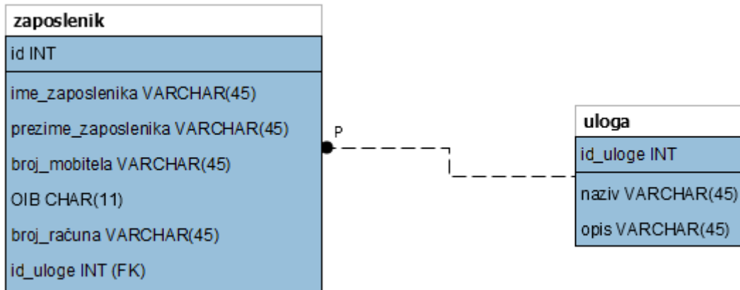
Slika 2.8 IDEF1X notacija
