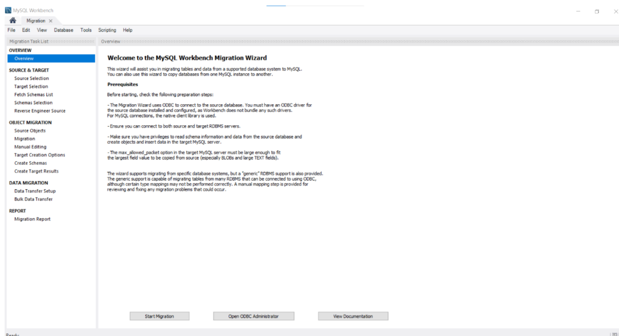
Slika 3.16 Premještanje podataka
