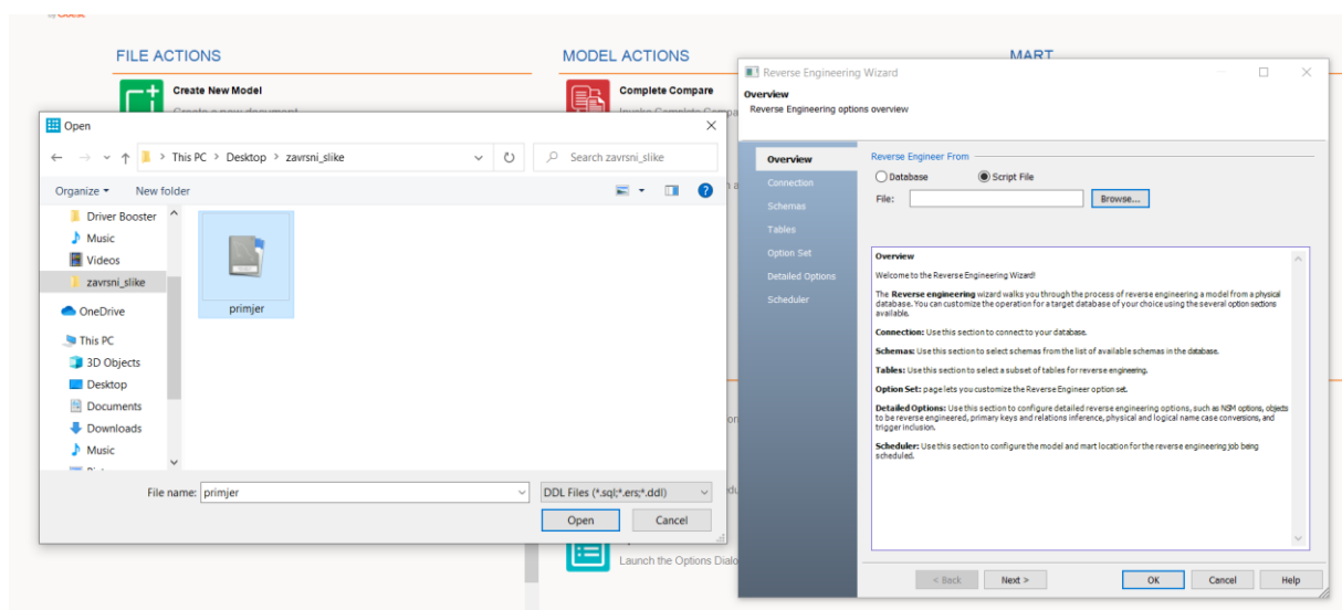
Slika 3.37 Odabir skripte
