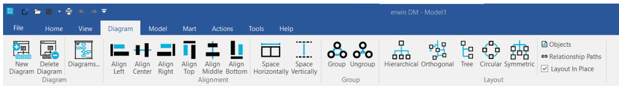
Slika 3.29 Erwin Diagram
