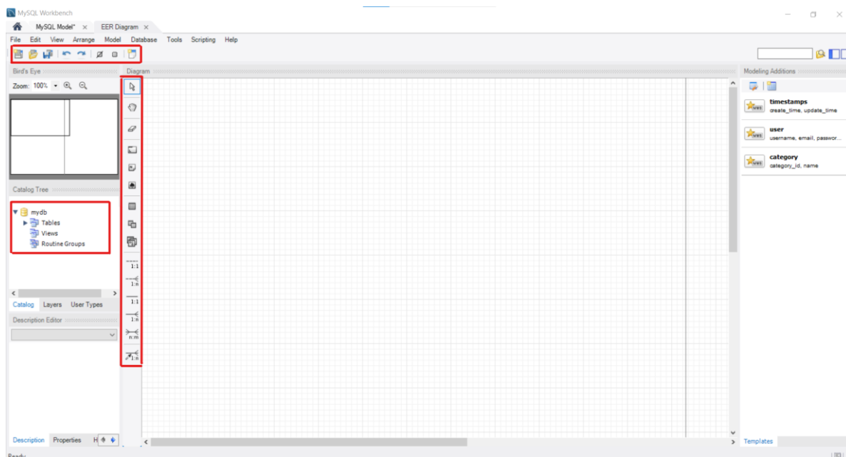
Slika 3.15 ERA dijagram
