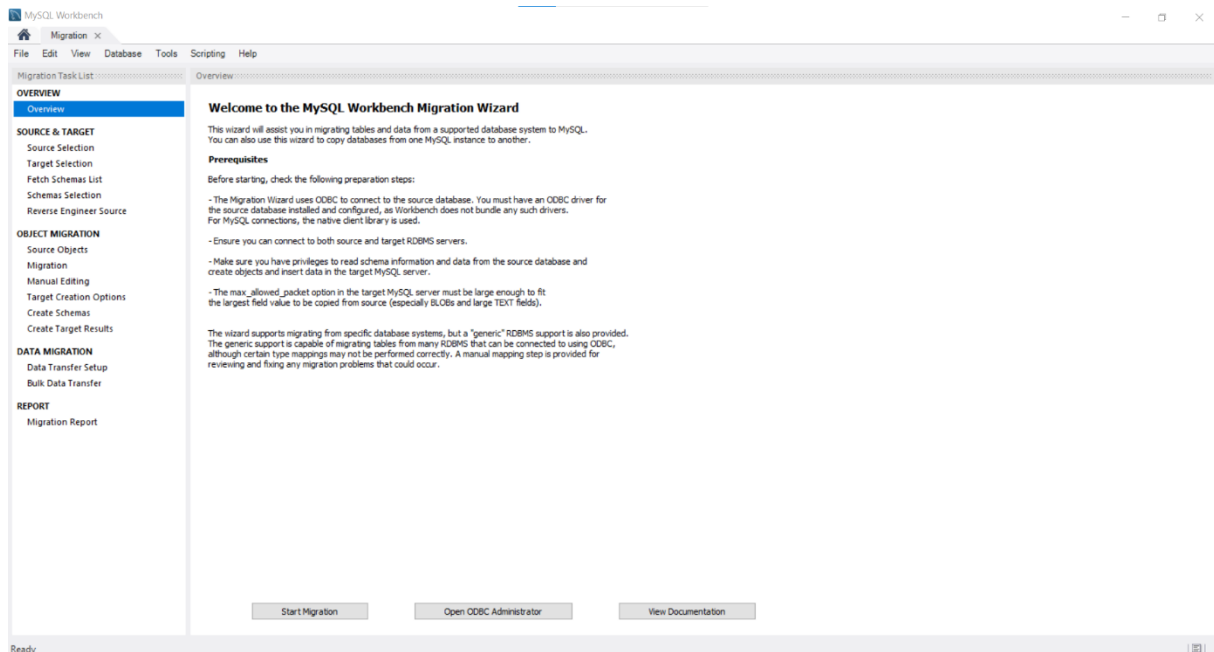
Slika 3.16 Premještanje podataka
