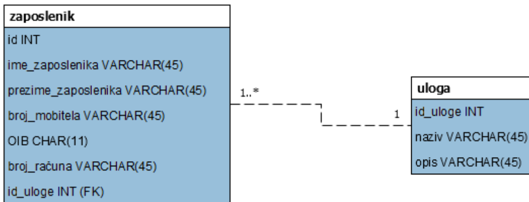
Slika 2.9 UML notacija
