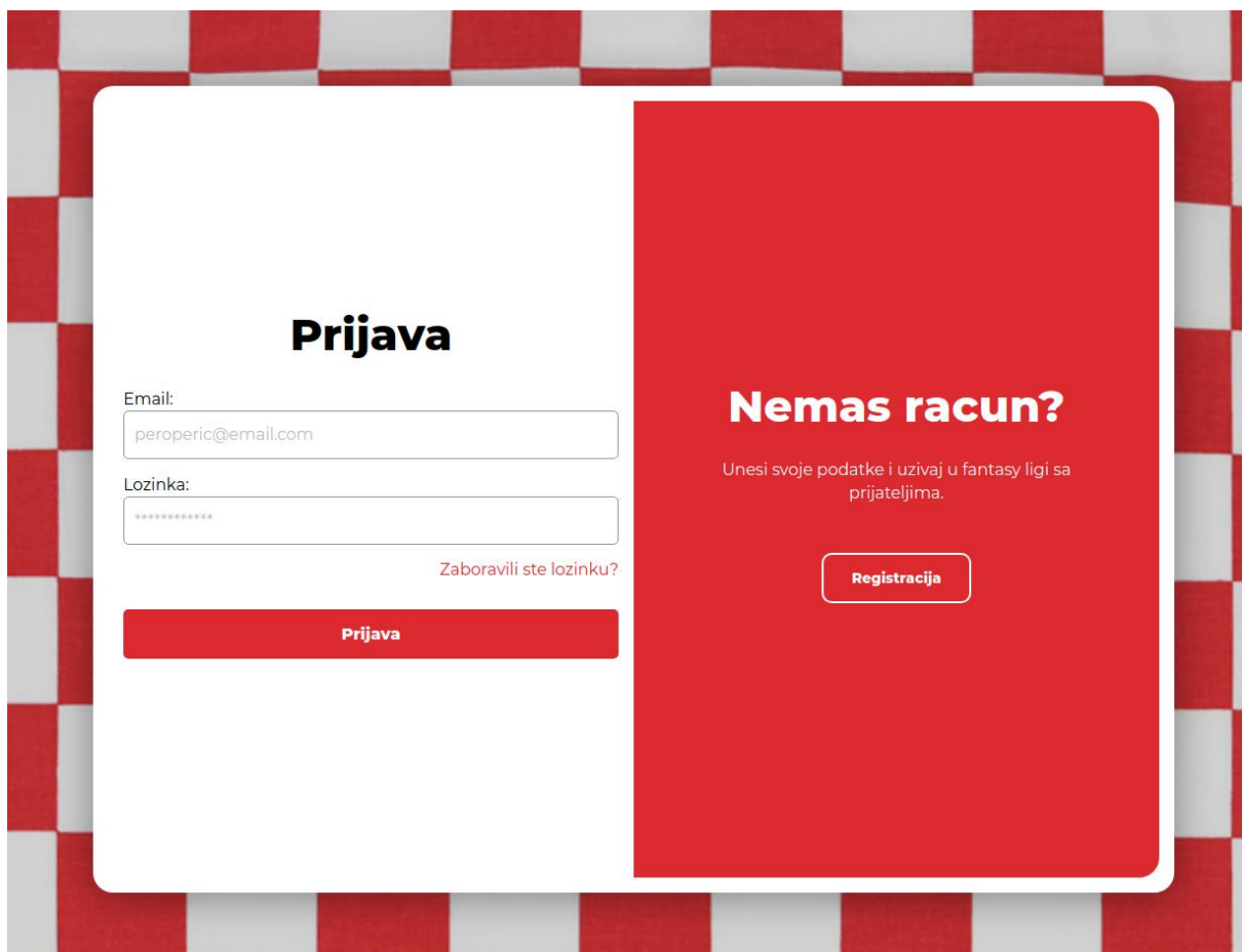
Slika 41: Autentikacija
