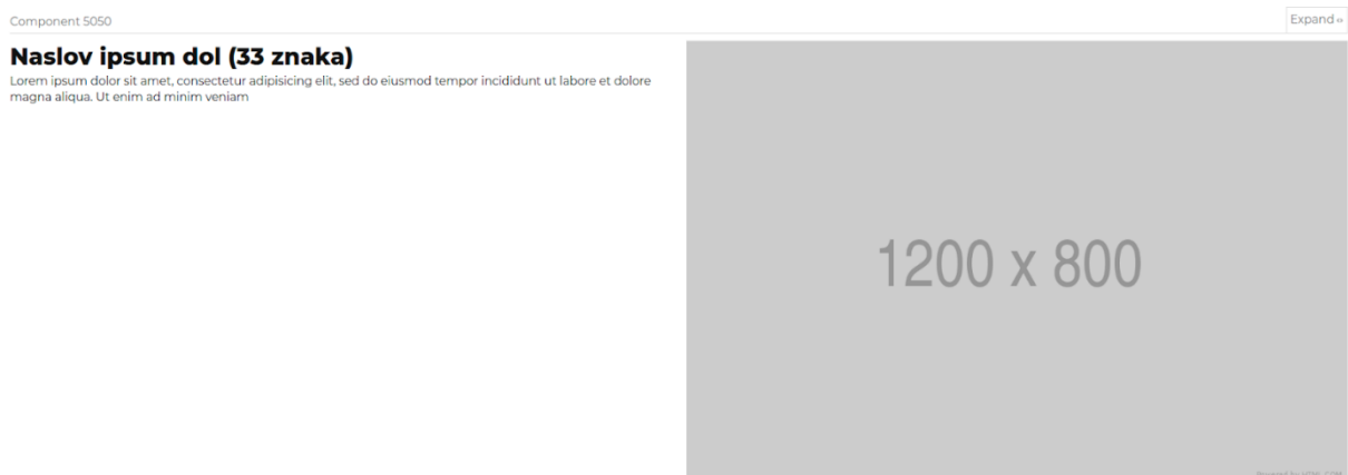
Slika 29: Molekula komponente 50-50
