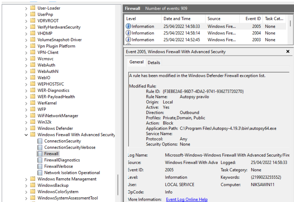
Slika 11.: Događaj izmjene postavki vatrozida za aplikaciju Autopsy (Izvor: Nikša Mirković, 2022)
