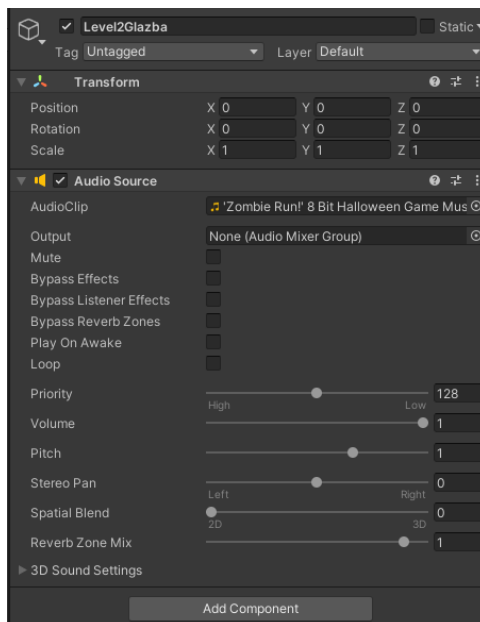
Slika 46: Primjer objekta sa komponentom „AudioSource“
