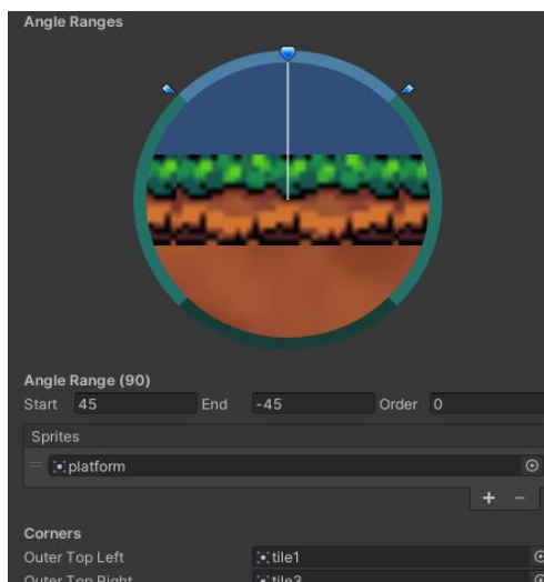
Slika 48: Komponenta „SpriteShape“
