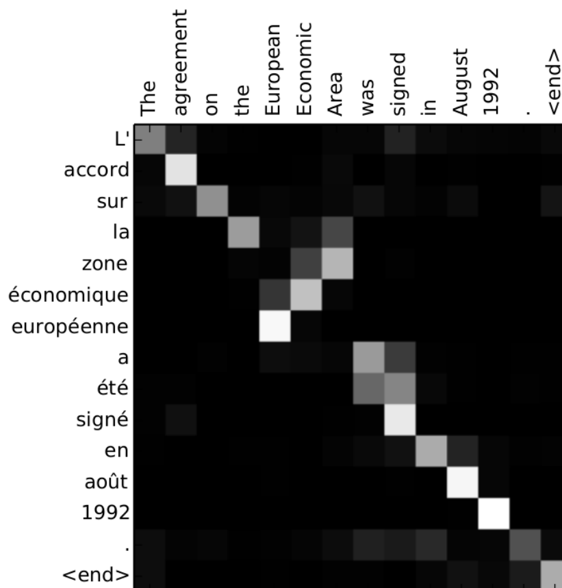
Slika 5: Kontekstualna ovisnost prilikom korištenja mehanizma pozornosti (Izvor: Bahdanau, Cho i Bengio, 2014)
