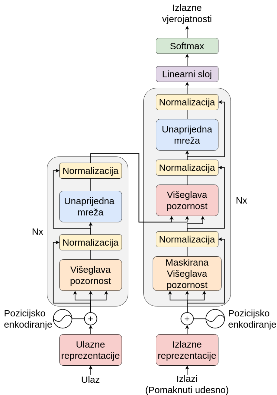
Slika 7: Arhitektura modela Transformer (Vlastita izrada prema: Vaswani, Shazeer, Parmar i dr., 2017)
