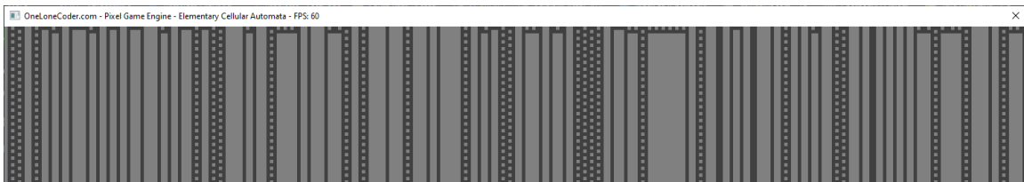
Slika 15: Pravilo 108 iz nasumičnog početnog stanja, Izvor: vlastita slika
