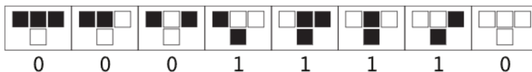
Slika 2: Grafički prikaz ishoda pravila 30 (00011110), Izvor: https://mathworld.wolfram.com/ElementaryCellularAutomaton.html
