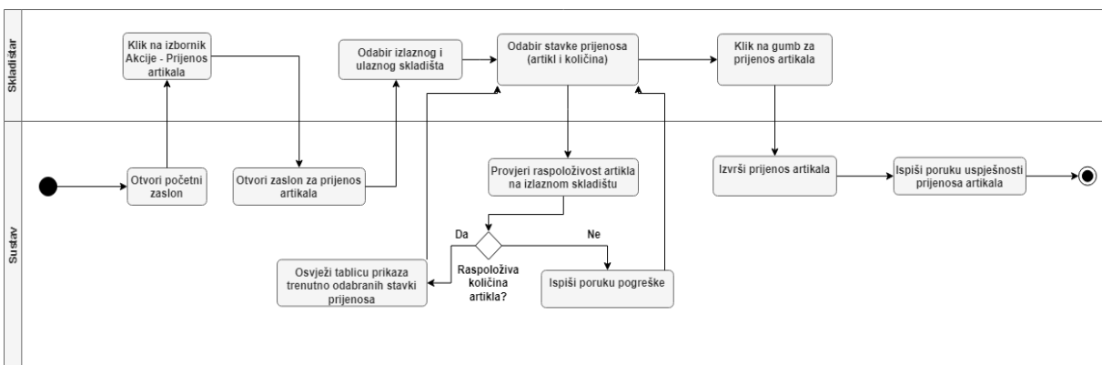
Slika 22. Dijagram aktivnosti prijenesa artikala između dva skladišta [autorski rad].
