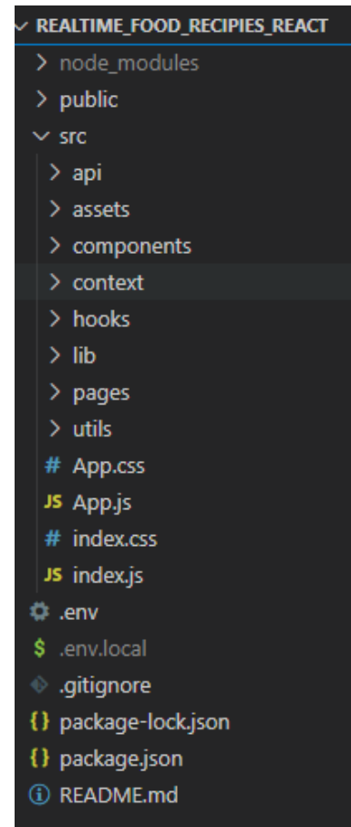
Slika 36: React struktura projekta
