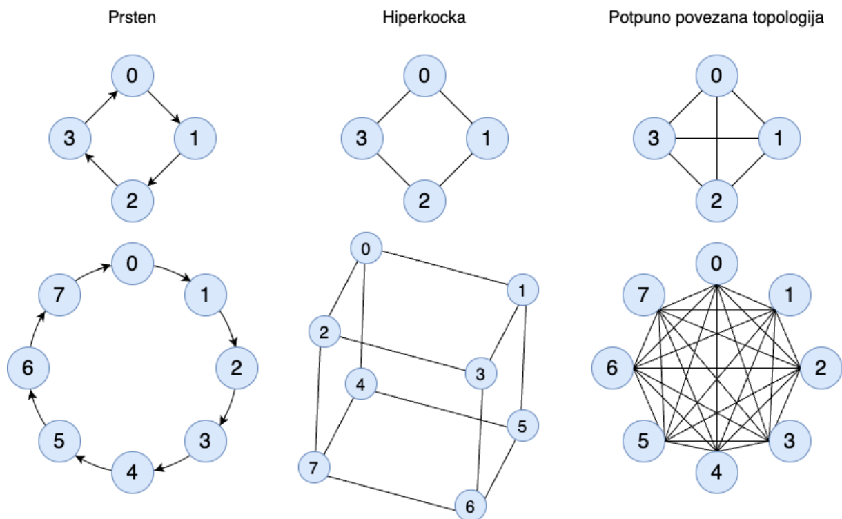
Slika 17. Komunikacijske topologije
