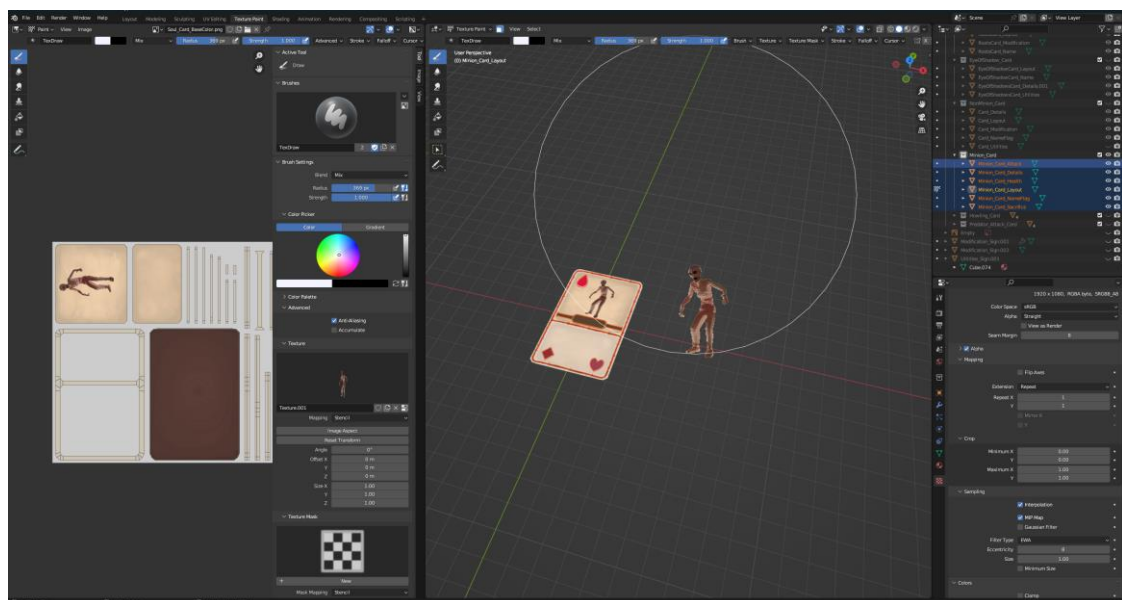
Slika 2. Blender sučelje
