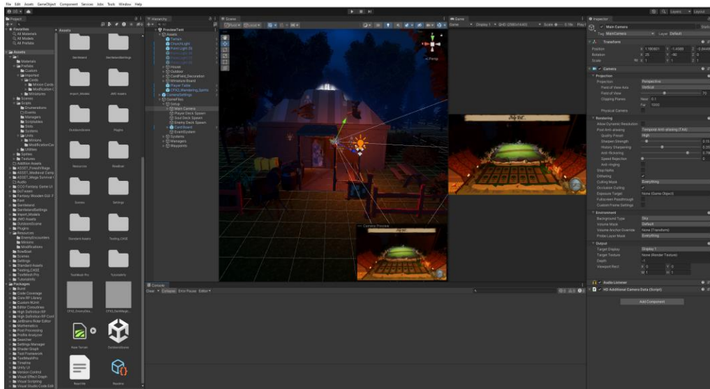
Slika 1. Unity sučelje
