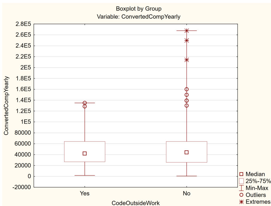
Slika 26: Dijagram s pravokutnicima za varijable CodeOutsideWork i ConvertedCompYearly (samostalna izrada)
