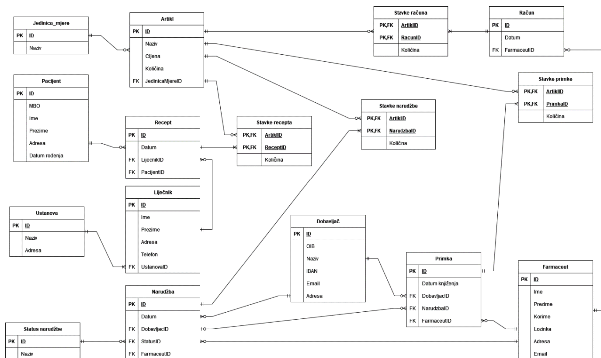
Slika 4: ERA model
