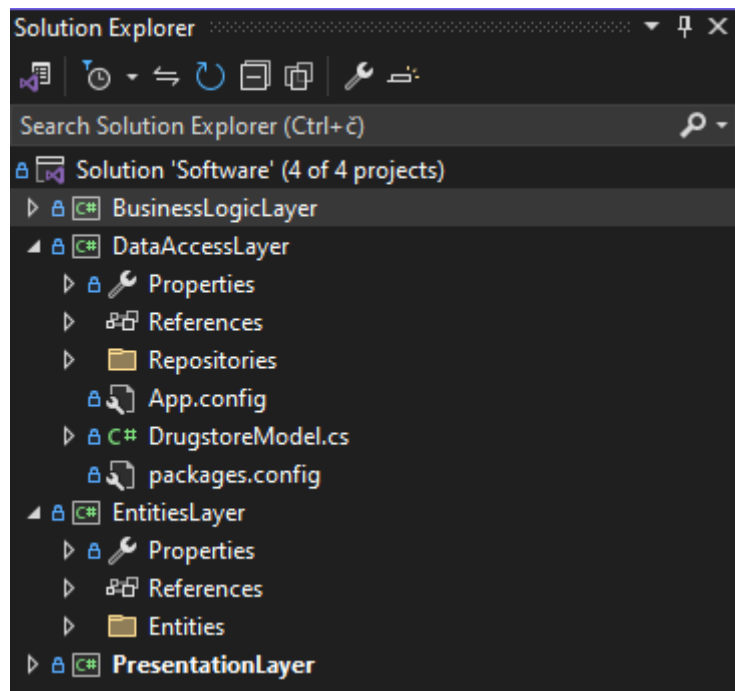
Slika 30: Struktura projekta
