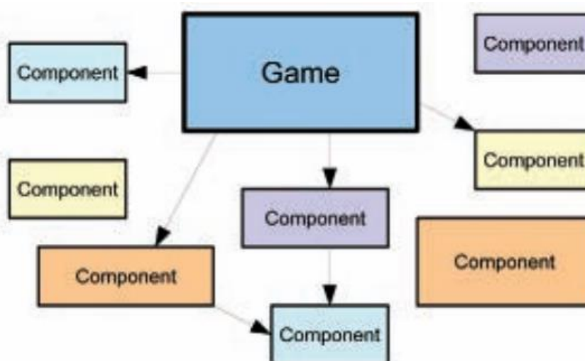
Slika 4. Toolkit arhitektura [6]
