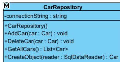
Slika 14: Dijagram klasa DataAccessLayer
