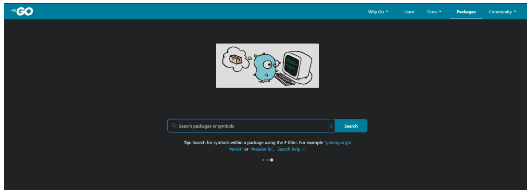
Slika 4. Prikaz go.dev-a
